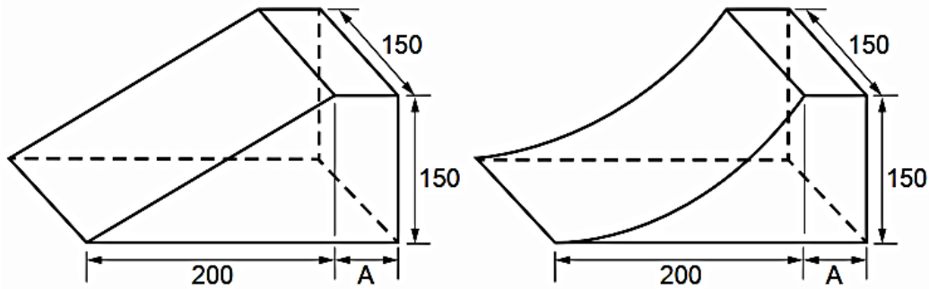
Modelo e dimensões dos calços em milímetros
